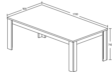
MODEL : DS 019-S5V ITEM : EETTAFEL / TABLE 170 / DINING TABLE 170 COLOR : NEW GREY OAK PRODUCT SIZE : L 170 X D 90 X H 76cm
