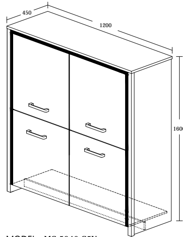
MODEL : MC 5046-S5V ITEM : ELIAS BAR 120 / 4 DOORS CABINET COLOR : NEW GREY OAK + BLACK LINE PRODUCT SIZE : L 120 x D 45 x H 160cm
