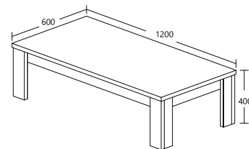
MODEL : CT 15035-S5V ITEM : SALONTAFEL / TABLE BASSE 120 / SOFA TABLE 120 COLOR : NEW GREY OAK PRODUCT SIZE : L 120 X D 60 X H40cm
