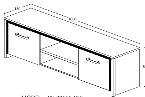
MODEL : EC 60155-S5V ITEM : ELIAS TV 160 / TV CABINET COLOR : NEW GREY OAK + BLACK LINE PRODUCT SIZE : L 160 x D 45 x H 55cm
