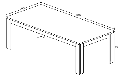
MODEL : DS 020-S5V ITEM : EETTAFEL / TABLE 190 / DINING TABLE 190 COLOR : NEW GREY OAK PRODUCT SIZE : L 190 X D 90 X H 76cm
